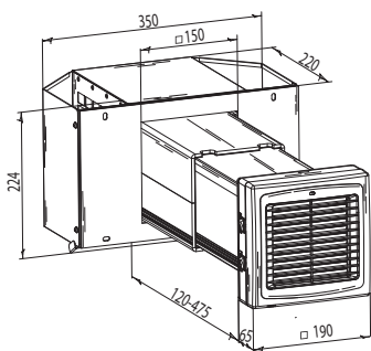
VENTO Ergo V50 S Pro
