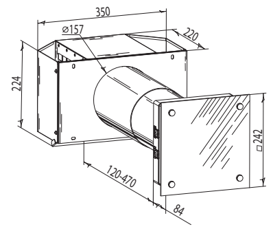
VENTO Ergo A50-1 S Pro
